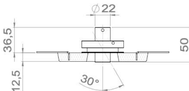
COUPE A-A ECHELLE 1 : 2
