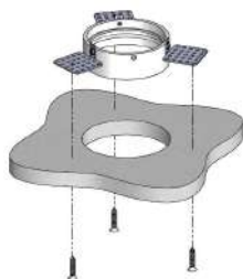
Principe d'installation par le dessus
