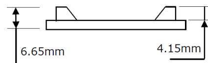
End cap
