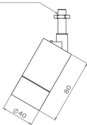
Tige filetée M10x1 + écrou
