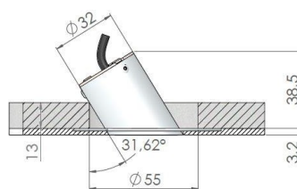
Double orientation 15°+ 29° (Version escalier)
